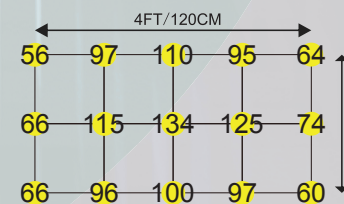
Height of 32"/ 80CM PAR Distribution
