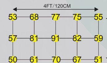
Height of 40"/ 100CM PAR Distribution
