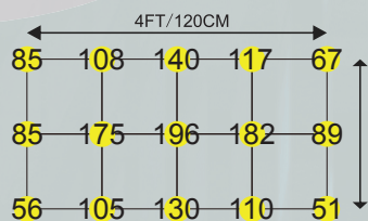
Height of 24"/ 60CM PAR Distribution
