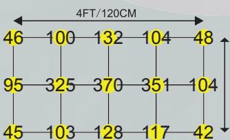
Height of 16"/ 40CM PAR Distribution
